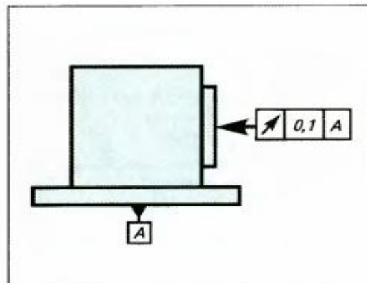
Рис. 17. Отклонение от перпендикулярности плоскостей
