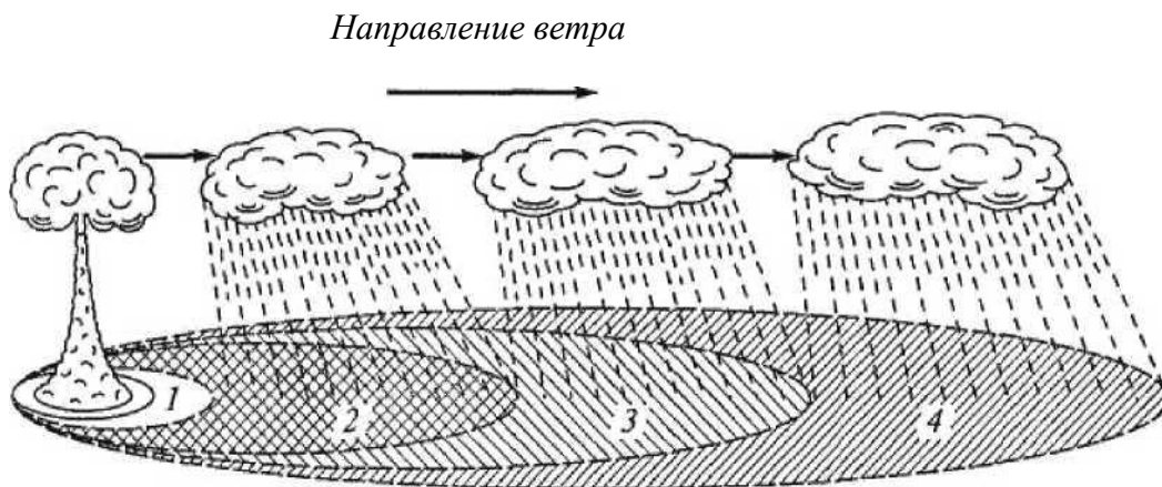
Рис. 5.2. Образование радиоактивного следа:
